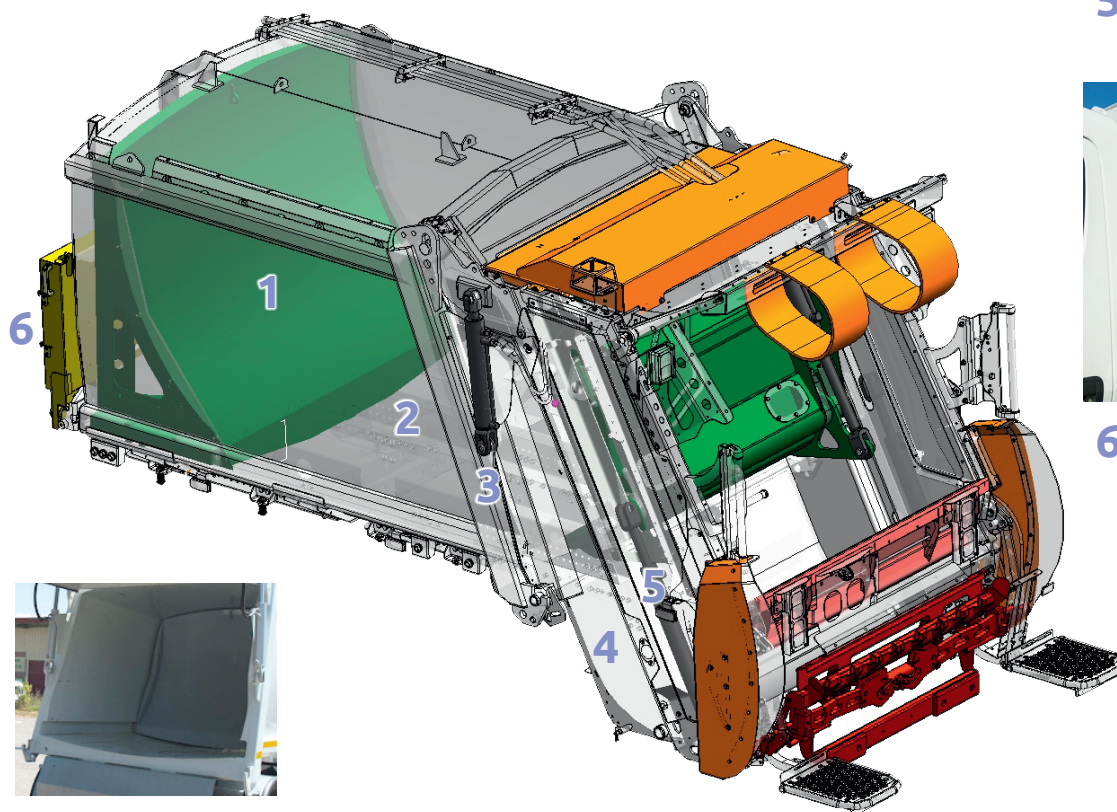
2 Kielvormige vloer met zijdelings geleiding voor het uitdrukschot.
